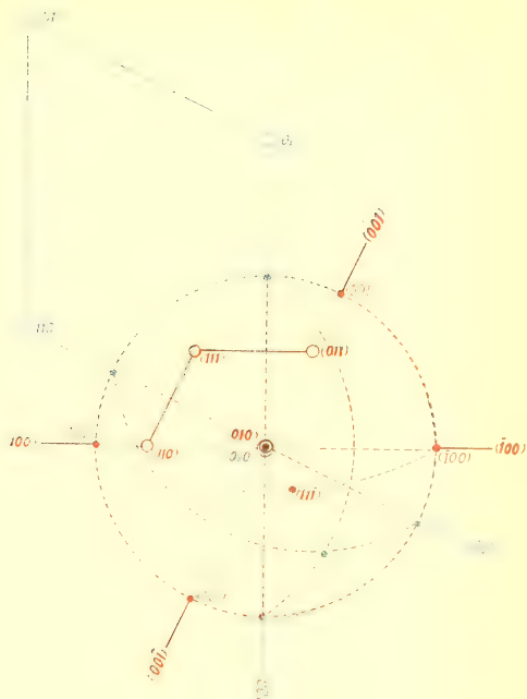
6. Двуплосный.
